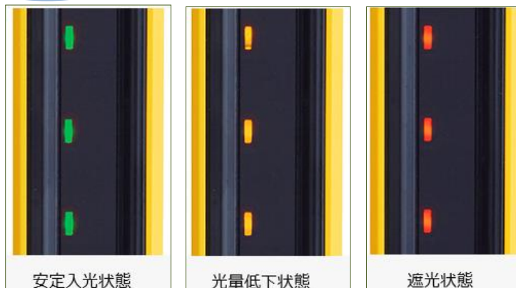
エリアビームインジゲータ(ABI)
